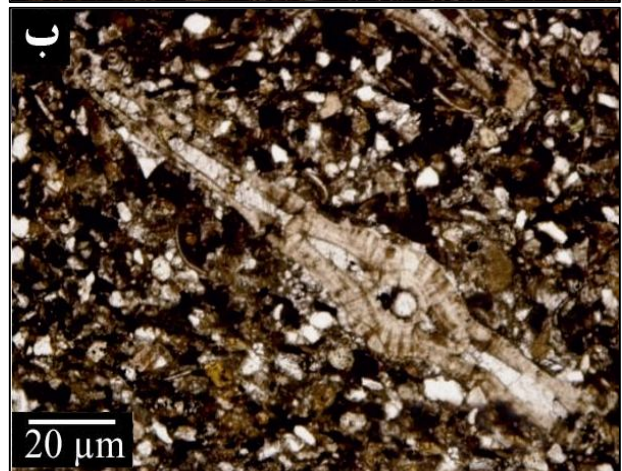
شکل ۵: الف) Operculina با دیواره ضخیم، بیانگر عمق کم و افزایش شدت نور (در مقطع B ۱۲ )؛ ب) Operculina با دیواره نازک، بیانگر عمق زیاد و کاهش شدت نور (در مقطع B ۱۶ )
