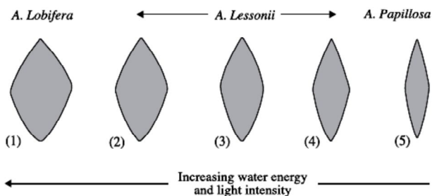
شکل ۷: تغییر در شکل و اندازه صدف Amphistegina در اثر تغییر میزان شدت نور و انرژی هیدرودینامیکی (Beavingtone-Penney & Racey, 2004)
