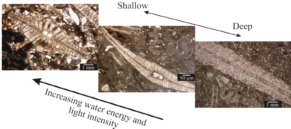
شکل ۸: تغییر در شکل و اندازه صدف در اثر تغییر در عمق، شدت نور و انرژی هیدرودینامیکی در جنس Lepidocyclina (از سمت چپ به راست درمقاطع نازک B ۲۷ , B ۲۱ و B ۲۱ )
