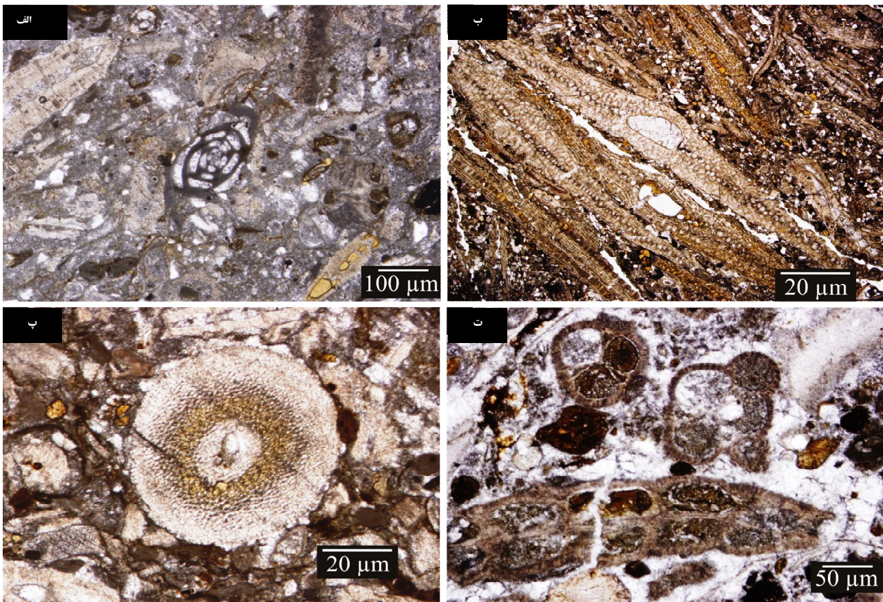
شکل ۹: الف: روزنداران منفردار به همراه روزنداران بدون منفذ ( B_8 تا B_{12} ); ب: روزنداران منفردار ( B_{13} تا B_{17} ); پ: اکتینید؛ ت: بریوزوا.
