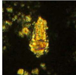
Nannocomus colomii
