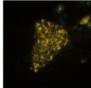
Nannocomus boletus
