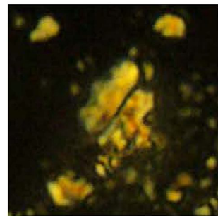
Nannoconus dolomiticus
