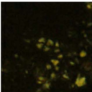
Watznaueria barnesae
