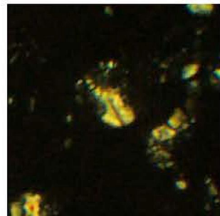
Nannoconus borealis
