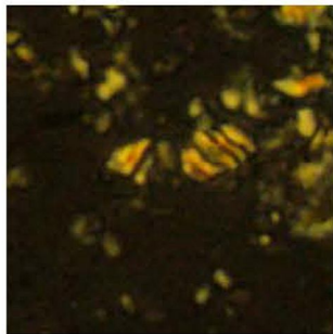
Comusphaera mexicana
