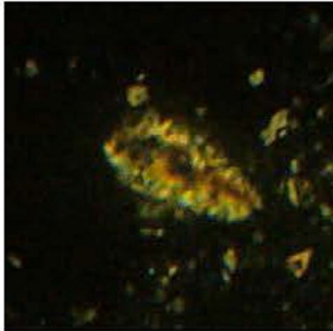
Nannocomus bermudezii
