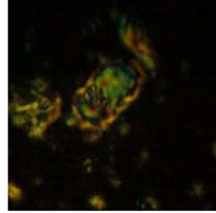
Nannoconus bucheri
