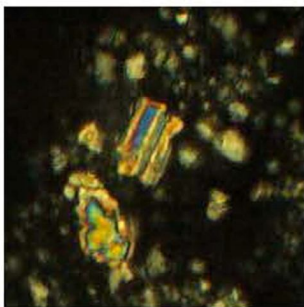
Nannoconus elongatus
