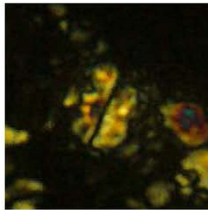
Nannoconus dolomiticus
