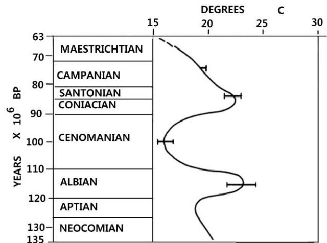
شکل ۲: منحنی دیرینه دمای کرتاسه شرق اروپا براساس ایزوتوپ O^{18} بلمنویدها (برگرفته از Urey et al., 1951؛ Lowenstam & Epstein, 1954؛ Bowen, 1961).
