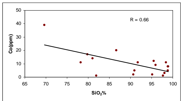
شکل ۱۰: ارتباط منفی بین Co و SiO 2
