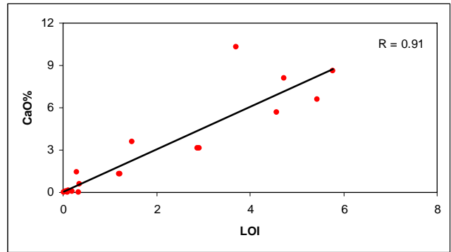
شکل ه الف: ارتباط مثبت بین LOI و CaO
