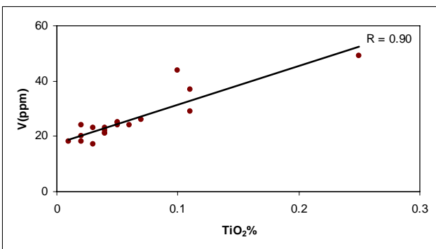
شکل ۱۱: ارتباط مثبت بین V و TiO 2
