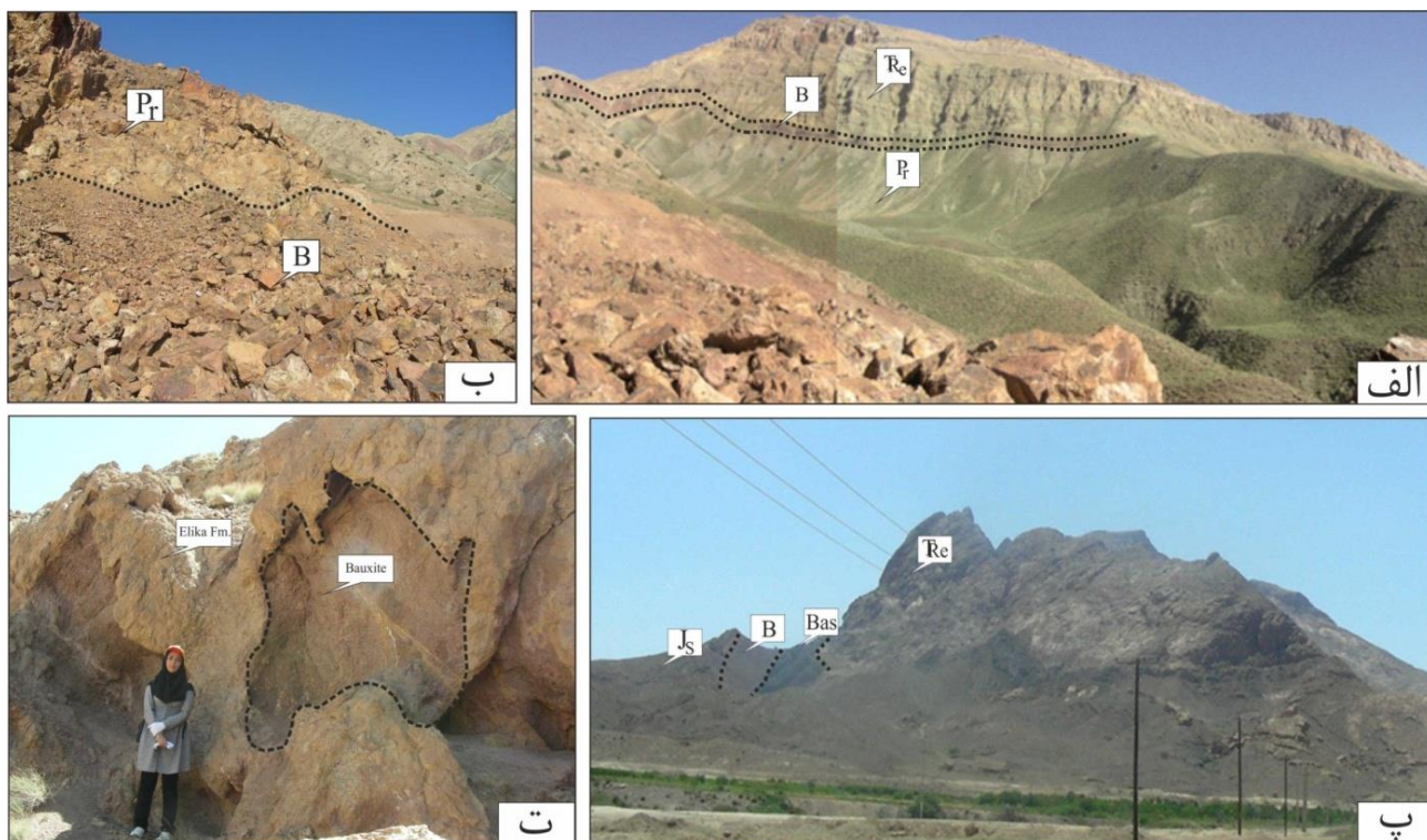
شکل ۲: تصاویر صحرایی از نهشته‌های تاش و آستانه؛ (الف) تظاهر لایه‌ای نهشته بوکسیتی تاش (نگاه به شرق)؛ (ب) مرز موج‌سان نهشته تاش با سنگ‌آهکهای سازند روته؛ (پ) نمای عمومی از منطقه آستانه؛ (ت) آکندگی حفرات کارستی سازند الیکا توسط مواد لاتریتی در نهشته آستانه (نشانه‌های اختصاری: B=افق بوکسیتی، Bas=بازالت، Js=ژوراسیک، سازند شمشک، Pr=پرمین، سازند روته، Re=تریاس، سازند الیکا).
