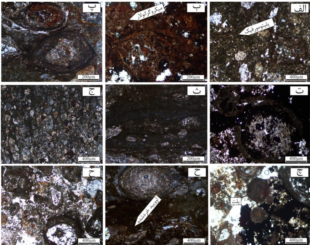
شکل ۴: تصاویر میکروسکوپی از شواهد بافتی برجازا و نابرجازا در نهشته‌های تاش و آستانه؛ الف) بافت پلیمورفیک؛ ب) بافت میکروگرانولار؛ پ) بافت اوئیدی؛ ت) بافت پیژوئیدی؛ ث) بافت جریانی - کلوفرمی؛ ج) بافت ریزآواری؛ چ) پلت؛ ح) اوئیدهای خردشده؛ خ) اوئیدهایی با اندازه و شکل متفاوت؛ همه تصاویر در نور گذرای عادی گرفته شده‌اند.
