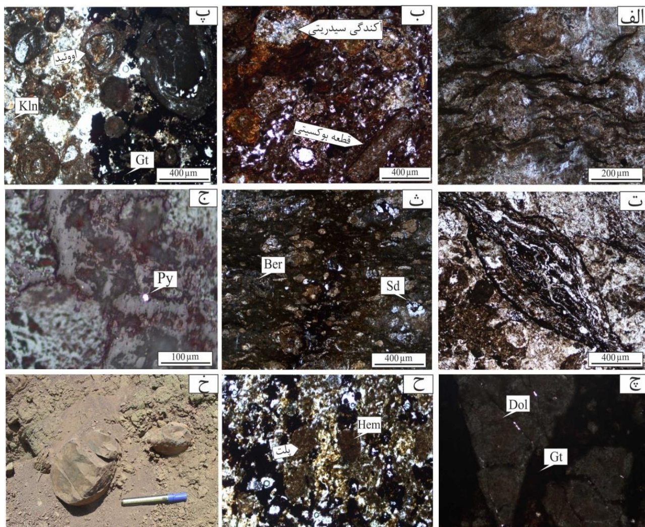
شکل ۶: تصاویر میکروسکوپی و ماکروسکوپی از واحدهای مختلف شناسایی شده در مناطق تاش و آستانه؛ الف) بافت جریان - کلوفرمی؛ ب) قطعات بوکسیت آواری در زمینه میکروگرانولار و آکندگی فضاها توسط کلسیت؛ پ) بافت اووئیدی؛ ت) اسپاستولیت؛ ث) قطعات بوکسیتی خرد شده با بافت ریزآواری؛ ج) پیریت افشان؛ چ) قطعات سنگی؛ ح) پلت‌های هماتیتی؛ خ) کنکرسینونهای واحد لاتریتی سبز آستانه (نشانه‌های اختصاری: Kln= کائولینیت، Sd= سیدریت، Ber= برتیرین، Py= پیریت، Dol= دولومیت، Gt= گوتیت، Hem= هماتیت). تصویر ج در نور بازتابی عادی و سایر تصاویر در نور گذاری عادی گرفته شده‌اند.
