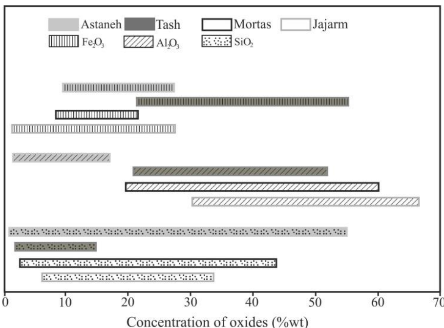
شکل ۸: تغییرات غلظت اکسیدهای Fe 2 O 3 , Al 2 O 3 و SiO 2 در نهشته‌های تاش و آستانه و مقایسه آن با کانسارهای جاجرم (امینی و همکاران، ۱۳۹۰؛ Mollai, 2011) و مورتاس (Öztrük et al., 2002).
