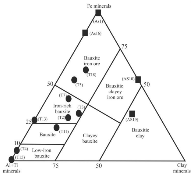
شکل ۷: مشخصات رخساره‌های نهشته‌های تاش (دایره توپر) و آستانه (مربع توپر) بر روی نمودار سه‌تایی کانیهای آلومینیوم - تیتان دار، کانیهای آهن دار و کانیهای رسی؛ برای مشخص شدن موقعیت صحرایی نمونه‌ها، شکل ۳ را ببینید (نمودار پایه از Bardossy, 1982).
