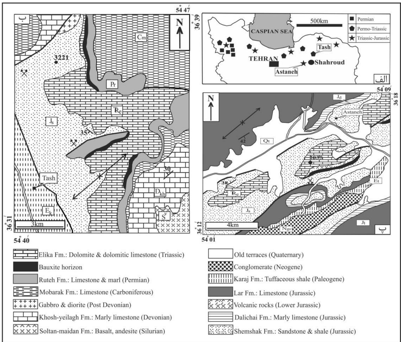
شکل ۱: الف) توزیع زمانی و مکانی نهشته‌های بوکسیتی در شمال ایران؛ در این شکل موقعیت جغرافیایی نهشته‌های تاش و آستانه نشان داده شده است. ب) نقشه زمین‌شناسی منطقه تاش؛ پ) نقشه زمین‌شناسی منطقه آستانه (نقشه پایه از شهرابی، ۱۳۶۹).
