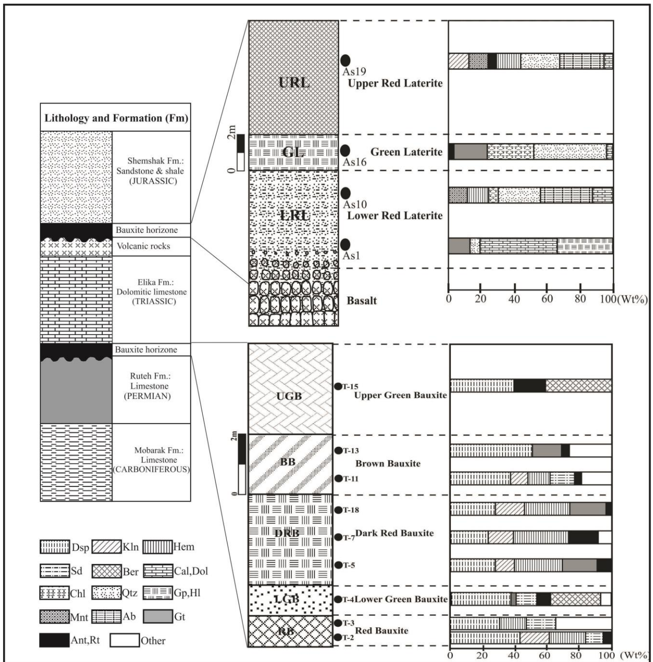
شکل ۳: توالی چینه‌شناسی طرح‌گونه از مناطق تاش و آستانه که در آن موقعیت چینه‌شناسی نهشته‌های مورد مطالعه مشخص شده است (سمت چپ). در این شکل تغییرات رخساره‌های نهشته‌های تاش (پایین) و آستانه (بالا) و نیز فراوانی نیمه‌کمی کانیها (سمت راست) نمایش داده شده است. دایره‌های توپر موقعیت نمونه‌برداری را نشان می‌دهند (نشانه‌های اختصاری: Dsp=دیاسپور، Kln=کائولینیت، Hem=هماتیت، Sd=سیدریت، Ber=برتیرین، Cal=کلسیت، Dol=دولومیت، Chl=کلریت، Qtz=کوارتز، Gp=ژپس، HI=هالیت، Mnt=مونتموریلونیت، Ab=آلبیت، Gt=گوتیت، Ant=آناتاز، Rt=روتیل، T=تاش، As=آستانه).
