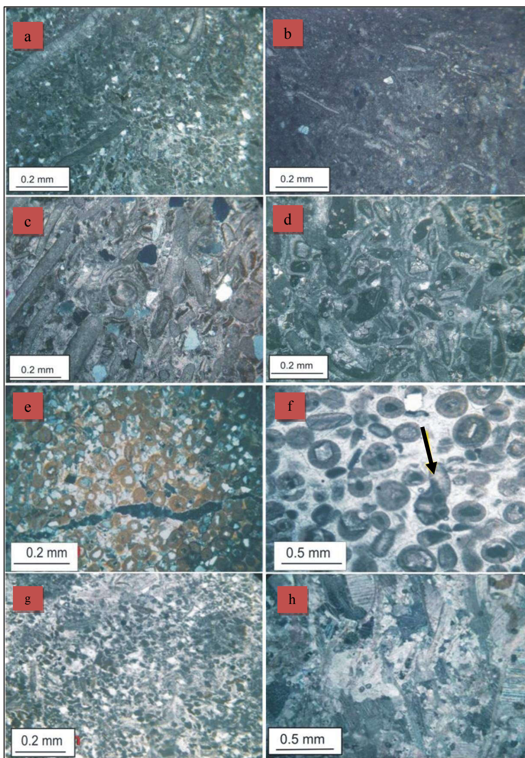
شکل ۴: a- پولیئیدال پکستون - وکستون (مقطع xpl، 48b). b- مادستون کوارتزی خرده فسیل‌دار (مقطع xpl، 34a). c- آنگال گرینستون ماسه‌دار (مقطع xpl، 51b). d- بایوکلاست پکستون - گرینستون ماسه‌دار (مقطع xpl، 44a). e- آئید گرینستون ماسه‌دار همراه با تخلخل کانالی. (مقطع xpl، 53b). f- آئید گرینستون، همراه با اینترکلاست (بیگان سیاه) و قطعات بایوکلاست (مقطع ppl، 56b). g- بایواینتراکلاست گرینستون (مقطع ppl، 48a). h- کریئوئید گرینستون، با قطعات بایوکلاست، احتمالاً دوکفه‌ایها (مقطع xpl، 59b).
