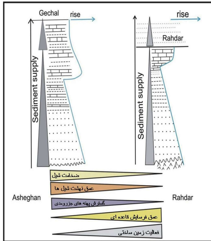
شکل ۱۳: مقایسه دو برش مورد مطالعه و بررسی تغییرات سطح آب دریا. در برش راهدار میزان فرسایش قاعده‌ای و زمین‌ساخت ناحیه‌ای نسبت به برش عاشقان فعالیت‌تر است. با وجود این، در برش عاشقان میزان ضخامت شیل و گسترش بیشتر پهنه‌های جزرومدی که در نتیجه فرونشست تدریجی به وجود آمده‌اند، فضای بیشتری برای نهشت این رسوبات ایجاد کرده است.
