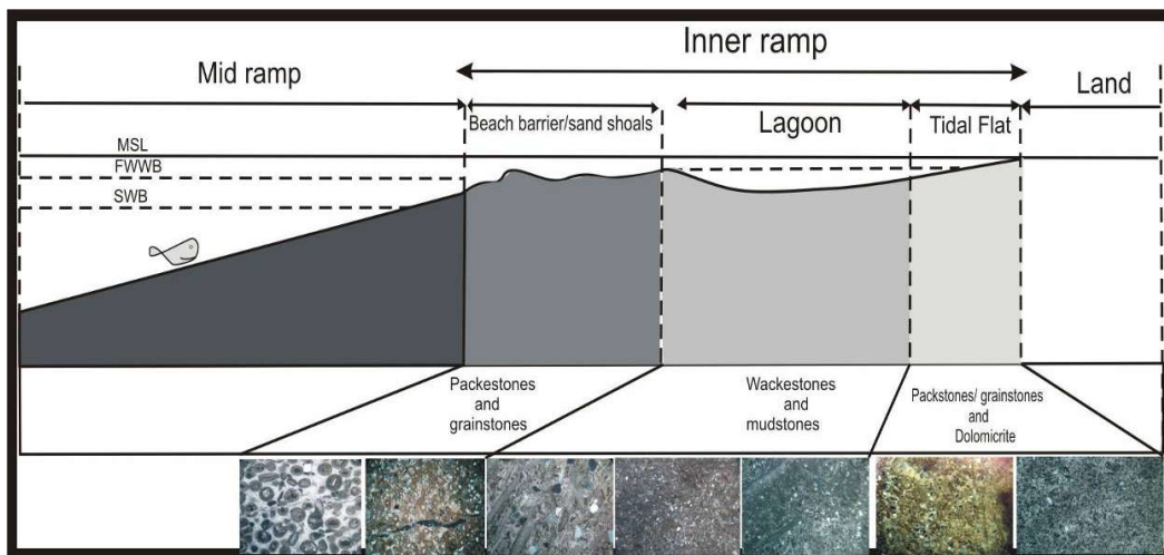
شکل ۱۲: مدل رسوبی کربناته سازند سازند شیرگشت. مدل سه بعدی نشان دهنده قسمت‌های مختلف یک رمپ است. مقطع عرضی، قسمت‌های مختلف رمپ داخلی کربناته‌های سازند شیرگشت را نشان می‌دهد.
