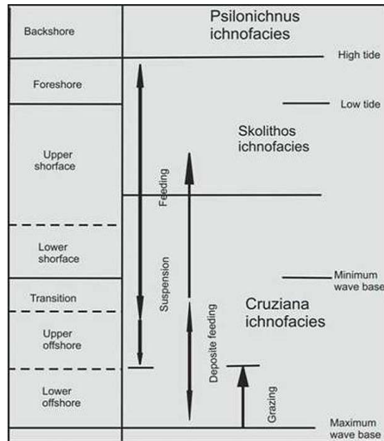
شکل ۷: مدل حاشیه ساحلی ایده‌آل ایکنوفاسیسیها بر اساس رفتار ارگانیسمها، عمق آب و سطح انرژی.
