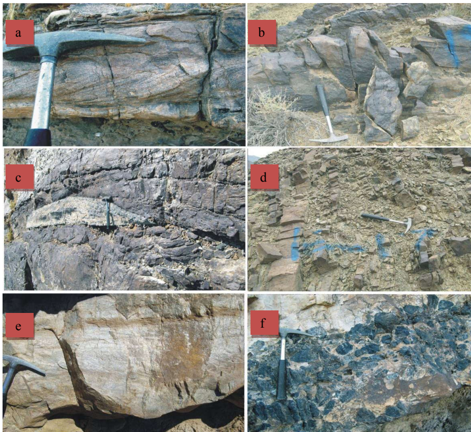
شکل ۸: a- ماسه‌سنگهای با طبقه‌بندی مورب مسطح در رخساره‌های Washover. b- ماسه‌سنگهای توده‌ای با آثار کروزیانا در رخساره Washover. c- آثار کانال جزرومدی در ماسه‌سنگها. d- شیل لامینه‌ای با میان لایه‌های ماسه‌سنگی. e- لایه‌های عدسی شکل طبقات کربناته در برش کوه راهدار. f- کنگلومرای چرتی سفید رنگ (الیگومکتیک) با پبلهای از نوع چرت و از نظر بافتی دارای جورشدگی و گردشگی خوب در بخش قاعده سازند شیرگشت در برش کوه عاشقان.
