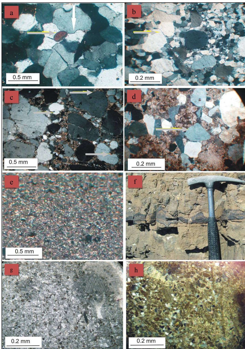
شکل ۳: a- جورشدگی خوب دانه‌های ماسه با تماس محدب - مقعر (پیکان سفید) و طولی، نقطه‌ای و دانه گرد شده گلوکونیت (پیکان خاکستری) (مقطع xpl، 28b). b- بایمودالیت در دانه‌های کوارتز همراه با تماس مضرس بین دانه‌های کوارتز (پیکان خاکستری) (مقطع 16a). c- فرورفتگی‌های خلیج مانند در دانه‌های کوارتز (پیکان خاکستری)، زمینه سنگ از سیمان دولومیتی (مقطع 31b). d- شکستگی دانه کوارتز (پیکان خاکستری) نشان از انرژی بالای محیط رسوبی، زمینه سنگ از سیمان دولومیتی. e- دولومیکرایت در پهنه جزرومدی (مقطع xpl، 28a). F- آثار ساخت استروماتولیت در دولومیتها (نشان دهنده پهنه‌های جزرومدی). g- بایوکلاست وکستون دولومیتی، همراه با قطعات کرینوئید (مقطع ppl، 31a). h- بایواینتراکلاست وکستون - پکستون (مقطع xpl، 42a).
