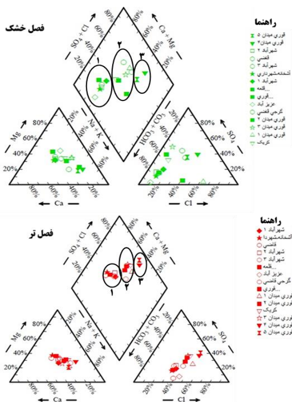
شکل ۵: نمودار پایپر نمونه‌ها
