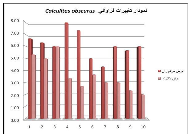
شکل ۱۰: نمودار فراوانی Calculites obscurus
