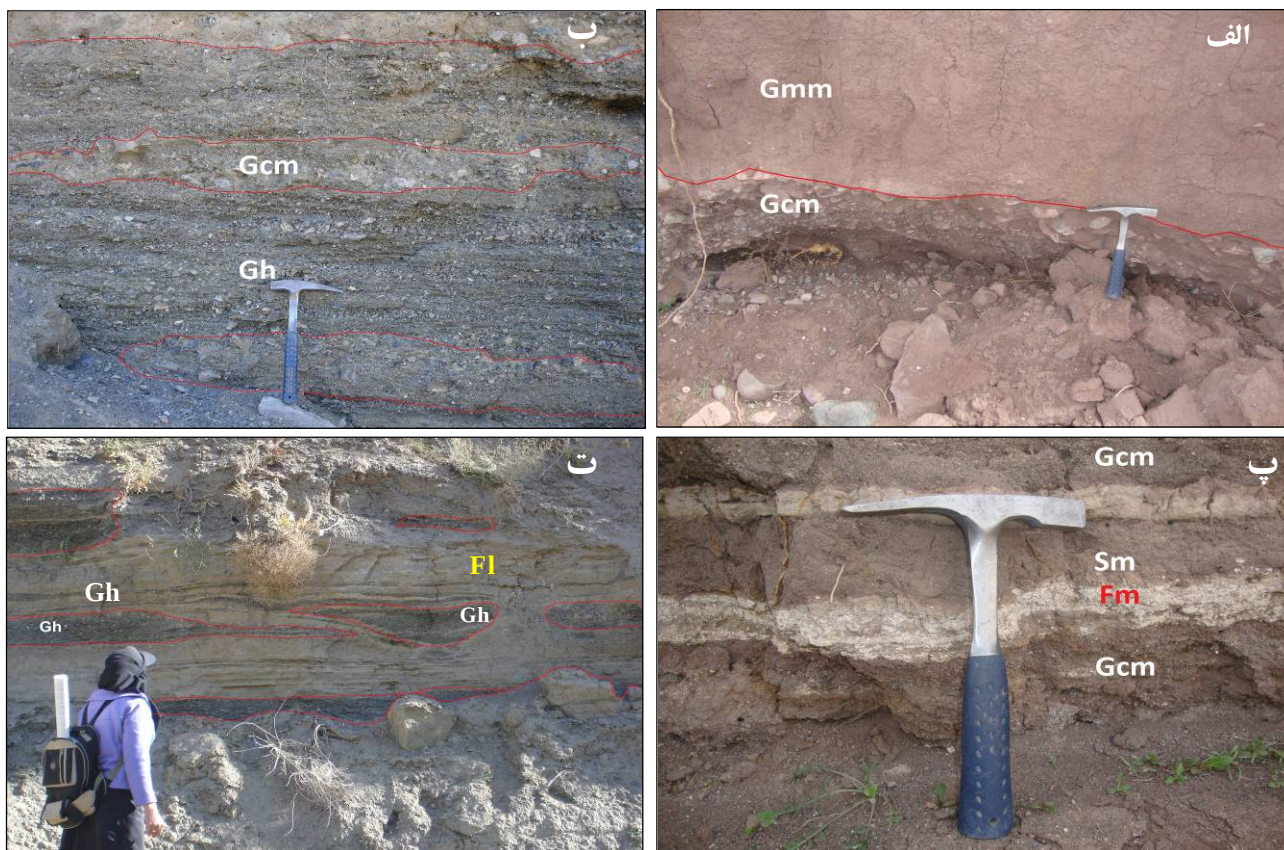
شکل 3: رخساره‌های رسوبی موجود در حوضه آبریز سرغایه - سرنیش: الف) رخساره‌های Gcm و Gmm (رودخانه سرغایه؛ ب) رخساره‌های Gcm و Gmm (رودخانه سرنیش؛ پ) رخساره‌های Gcm، Gmm، Gh و Fm (رودخانه سرنیش؛ ت) رخساره‌های Gcm، Sm، Fm و Gh (رودخانه سرغایه؛ پ) رخساره‌های Gcm و Gmm (رودخانه سرنیش؛ پ)
