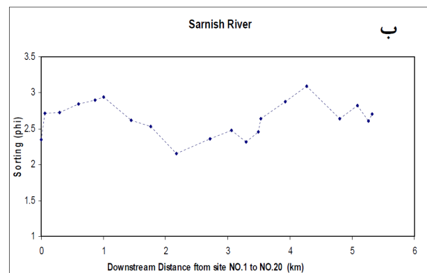
شکل 9: تغییرات جورشدگی اندازه ذرات از بالادست به سمت پایین دست (الف) رودخانه سرغایه و (ب) رودخانه سرنیش
