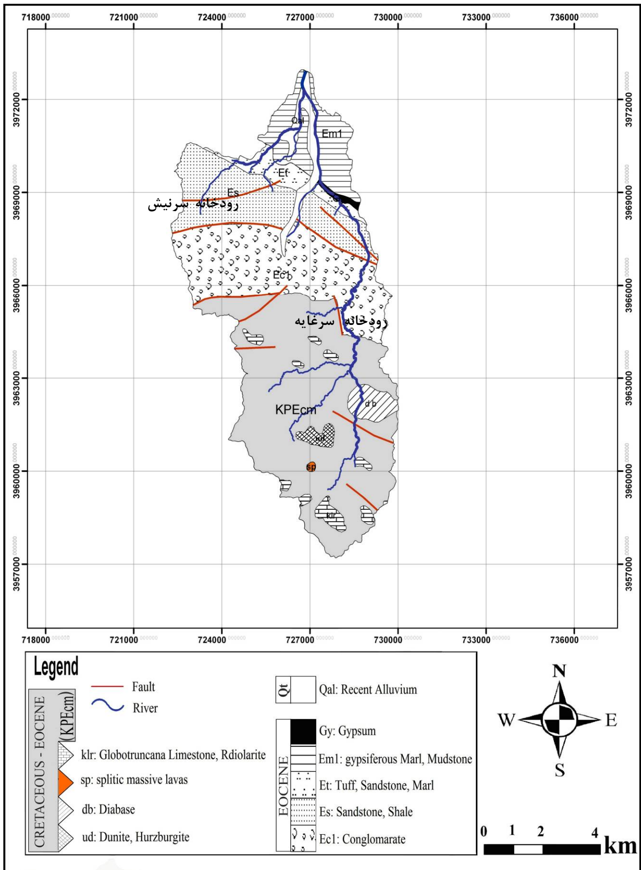
شکل 2: نقشه زمین شناسی حوضه آبریز سرغایه - سرینیش با استفاده از نقشه 1:250000 تربت حیدریه (واعظی پور و همکاران، 1370)
