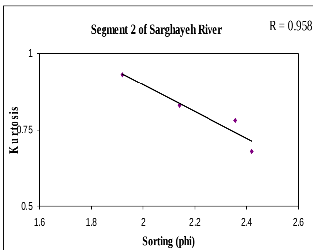
شکل 12: رابطه بین ضریب جورشدگی و کشیدگی در طول رودخانه سرغایه
