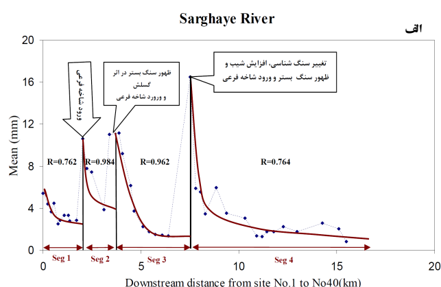
شکل 4: الف) تغییرات میانگین ذرات به طرف پایین دست رودخانه سرغابه
