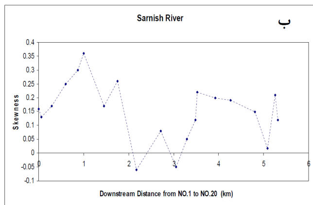
شکل 10: تغییرات کج شدگی اندازه ذرات از بالادست به سمت پایین دست (الف) رودخانه سرغایه و (ب) رودخانه سرنیش
