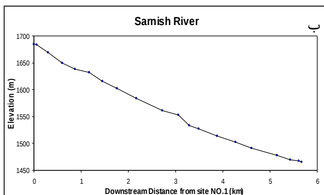
شکل 5: الف) پروفیل طولی رودخانه سرغابه و ب) پروفیل طولی رودخانه سرنیش از بالادست به سمت پایین دست بر اساس محلهای نمونه برداری
