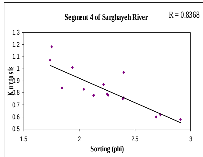
ادامه شکل 12: رابطه بین ضریب جورشدگی و کشیدگی در طول رودخانه سرغایه
