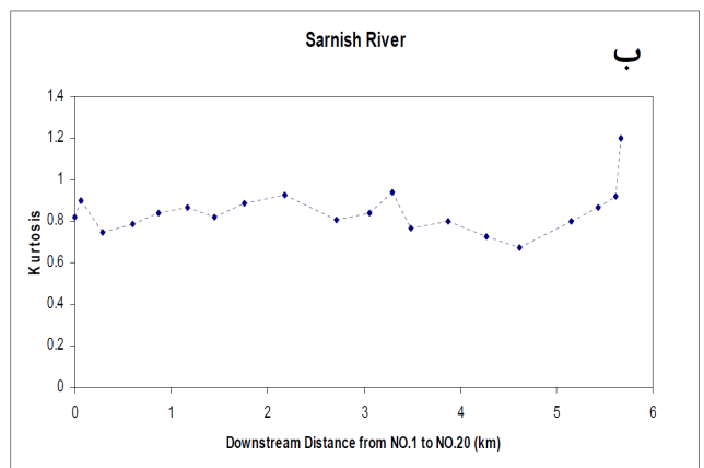
شکل 11: تغییرات کشیدگی اندازه ذرات از بالادست به سمت پایین دست (الف) رودخانه سرغایه و (ب) رودخانه سرنیش
